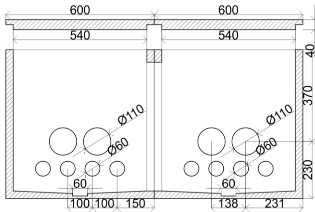
CORTE A-A'
