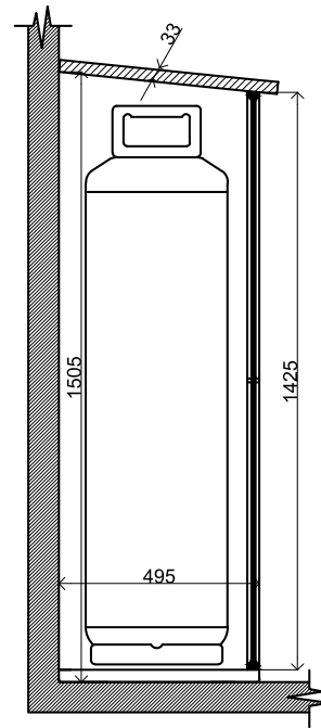
CORTE
