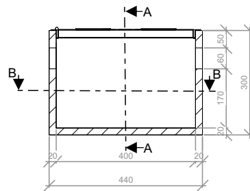
PLANTA
