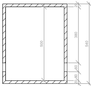
CORTE B-B
