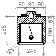
CORTE B-B
