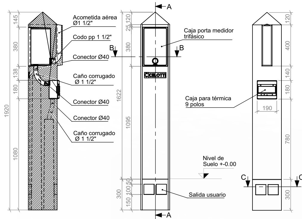
CORTE A-A
