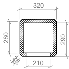
CORTE B-B
