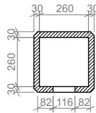
CORTE C-C
